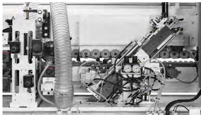
前后切单元：配备了高精度直线导轨的坚固结构保证了前后切精度
