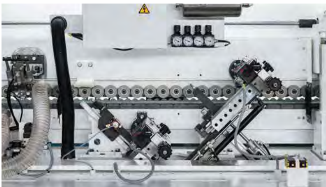
跟踪导圆单元：可以加工厚PVC边带，工件厚度最大60毫米。速度16米/分钟
